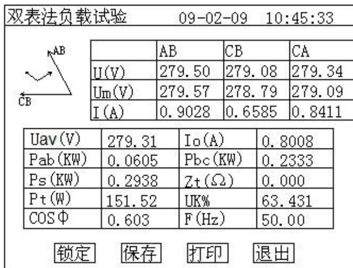
图 11 负载试验测试数据页面
