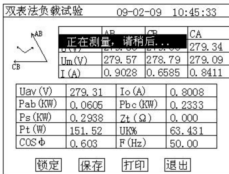
图 12 负载损耗正在测量计算页面
